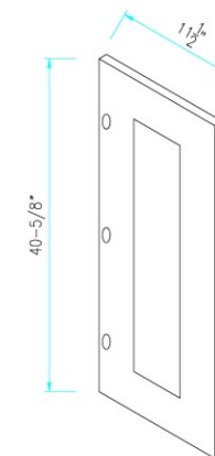
DUMMY DOOR W1242
