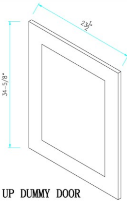
DOOR W3630 DUMMY DOOR B36
